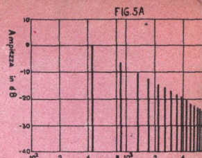
Fig. 5 - La figura superiore rappresenta lo spettro di frequenza di un'onda a denti di sega della (frequenza) fondamentale di 440 Hz. Nelle figure inferiori di sinistra e di destra lo stesso spettro della frequenza modificato dopo il passaggio rispettivamente attraverso filtri passa-alto e passa-basso.
