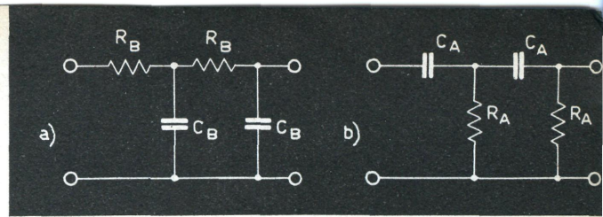
Fig. 3 - Filtri a resistenza e capacità.
