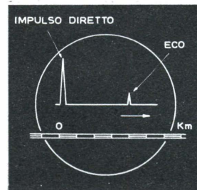
Fig. 4 - Principio di misura su schermo oscillografico.
