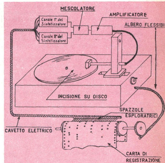
Fig. 7 - La serie delle spazzole esploratrici, passando sui fori delle carte di registrazione, predispone nel sintetizzatore i vari circuiti per la generazione di due distinti ed indipendenti segnali di uscita: Canale 1° e Canale 2° che nel mescolatore danno luogo ad un segnale risultante adeguatamente amplificato prima di comandare il registratore.
