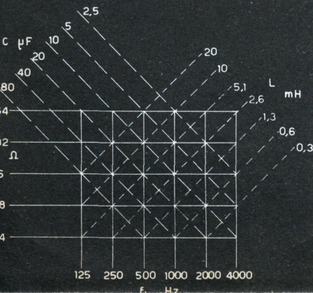
Fig. 2 - Abaco per il calcolo dei filtri di fig. 1.
