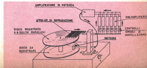
Fig. 8 - 16 pick-up esplorano il disco a 6 solchi paralleli; le relative uscite, i cui livelli possono essere singolarmente regolabili, vengono preventivamente amplificate. Il segnale risultante entra nell'amplificatore di potenza prima di iniziare l'incisione del disco inferiore nello schema qui sotto.
