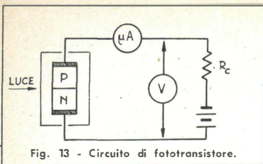
Fig. 13 - Circuito di fototransistore.
