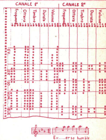
Fig. 6 - Carta di registrazione a perforazione del sintetizzatore a due canali indipendenti. La frase EVER SO HUMBLE, registrata con questo sistema, è stata ripetuta in basso con le notazioni convenzionali. L'allineamento dei fori superiori punzonati a solo titolo di riferimento dà l'indicazione del numero di combinazioni, secondo il sistema binario, assegnato ad ognuna delle caratteristiche del suono per la segnalazione di tutti i circuiti interessati.
