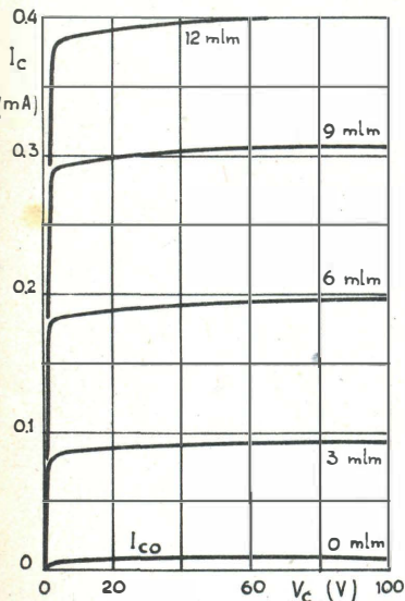
Fig. 15 - Caratteristica di fototransistore a giunzione.
