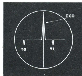
Fig. 6 - Presentazione parziale per indicazione di precisione.
