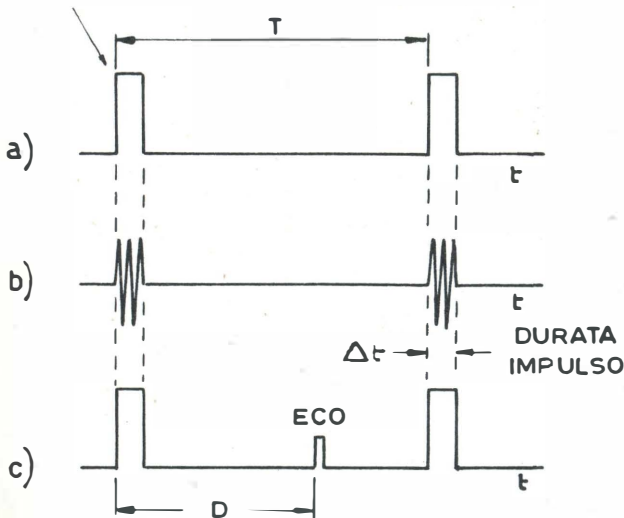
Fig. 3 - Impulsi di funzionamento.
