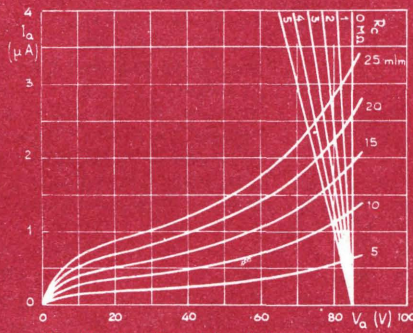
Fig. 7 - Caratteristiche di fototubo a gas.
