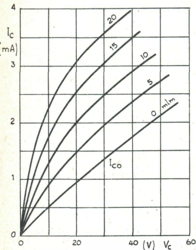
Fig. 14 - Caratteristiche di fototransistore a punta.
