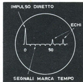
Fig. 5 - Scala oscillografo radar lineare (scansione tipo A).
