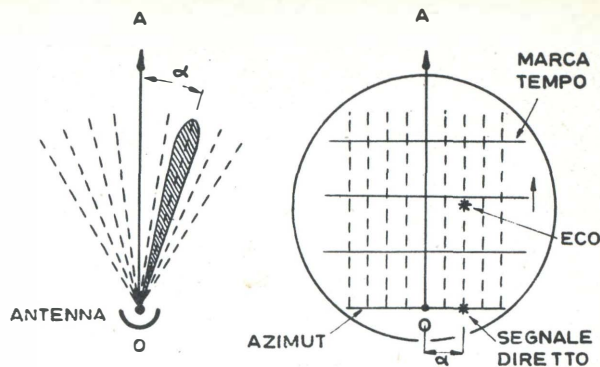
Fig. 8 - Esplorazione radar di tipo B.
