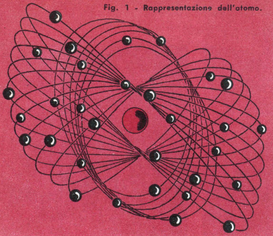
Fig. 1 - Rappresentazione dell'atomo.
