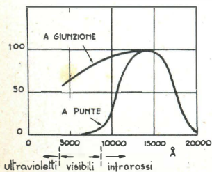
Fig. 16 - Caratteristica di sensibilità di fototransistori.
