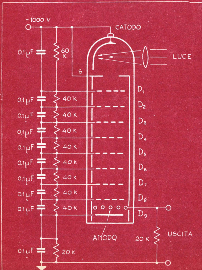
Fig. 9 - Connessione di fotomoltiplicatori.
